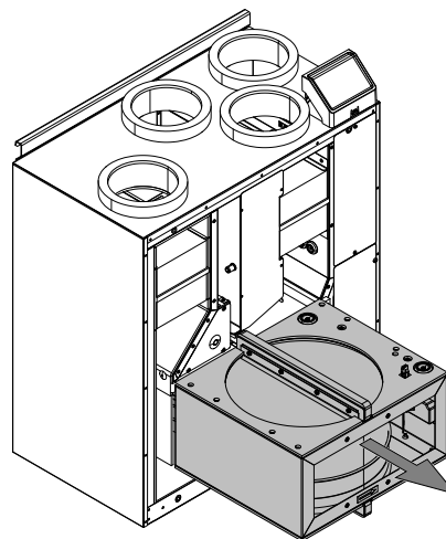
Fig. 5 Värmeväxlare
