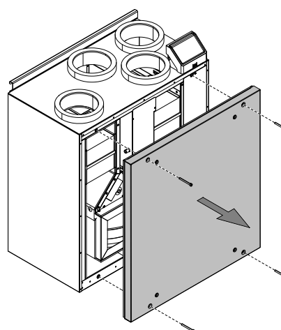
Fig. 3 Demontering/montering av invändig front
